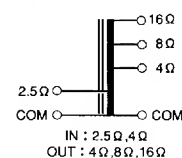
回路図 CIRCUIT
