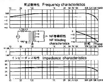
F-2011 特性表
