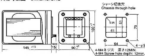
外形寸法図 DIMENSIONS
